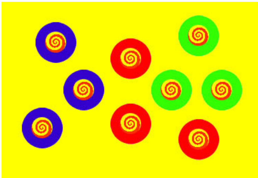
Рисунок 5. Монады
