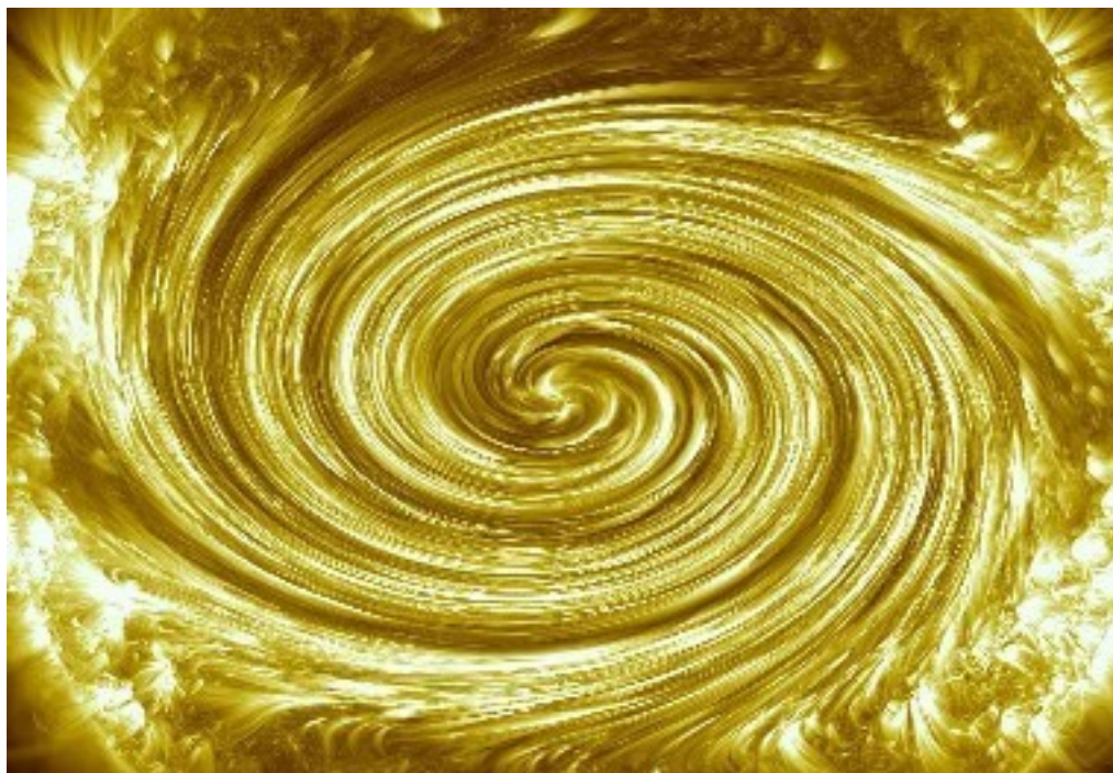
Рисунок 3. Глубины монады
