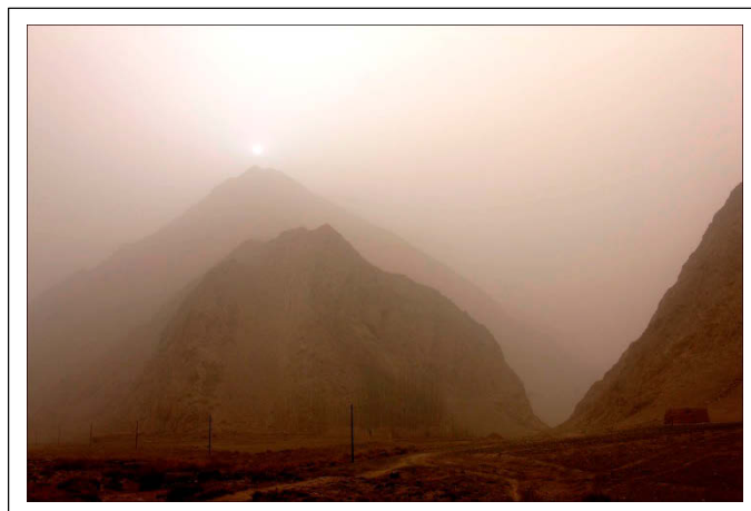
Такла-Макан. Пыльная буря. (Современное фото)
